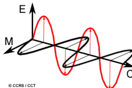
Obrázek 2 Elektromagnetické záření
