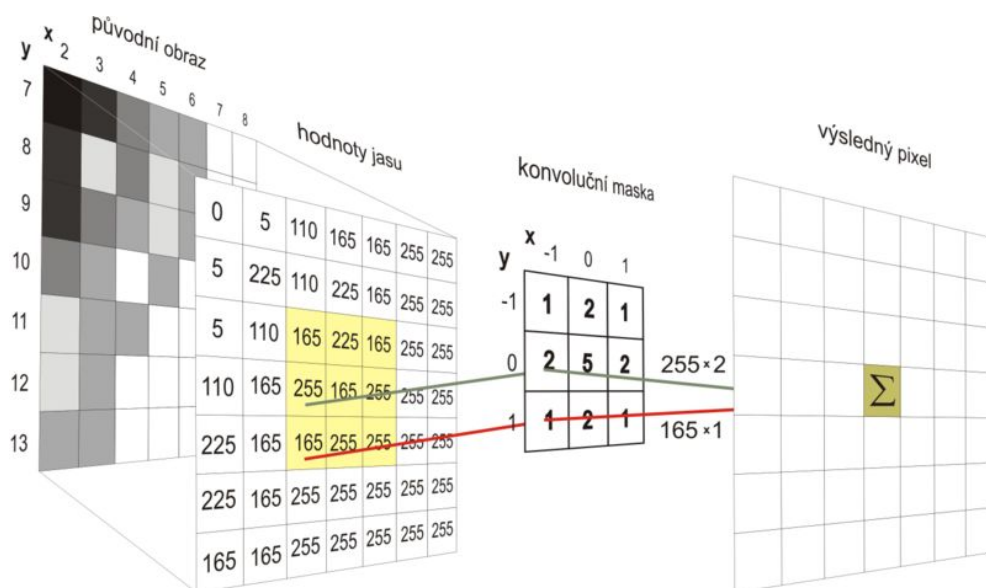
Obrázek 17 Princip konvoluce
