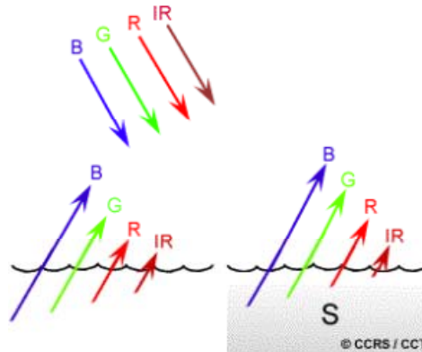
Obrázek 8 Odrazivost vody
